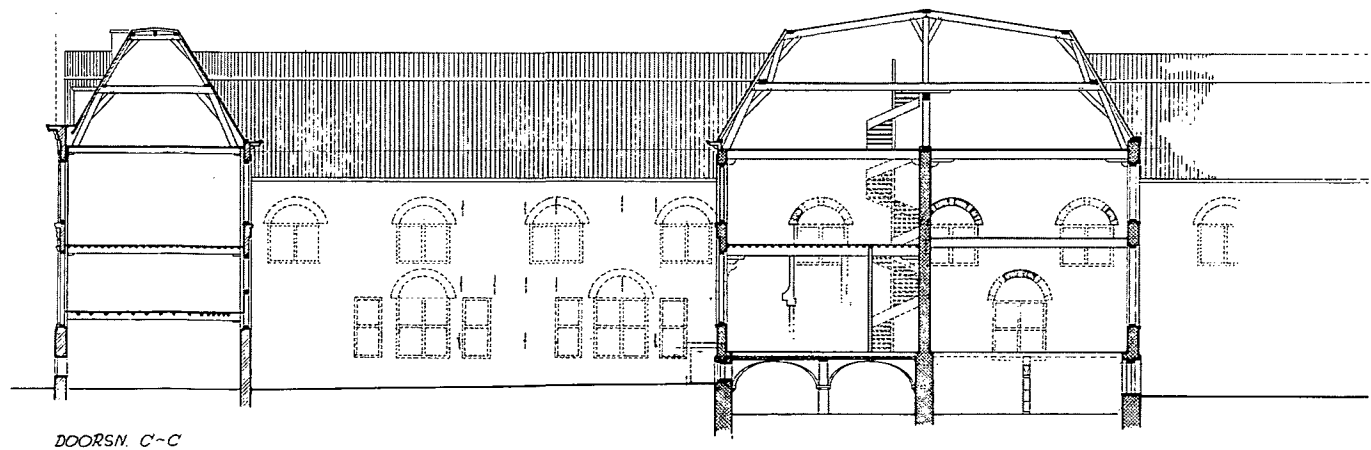
Afb. 6. Amsterdam, het v.m. Oost-Indisch huis, Oude Hoogstraat 24. Dwarsdoorsnede van het poortgebouw aan de Oude Hoogstraat en van de zuidvleugel gezien in oostelijke richting naar het v.m. Bushuis. Proeve van een reconstructie van de bestaande toestand in 1890 naar opmeting van het architectenbureau Bart van Kasteel en J. Schipper in 1975 en tekeningen van C.H. Peeters in 1890 (tekening J.J. Jehee 1978).
