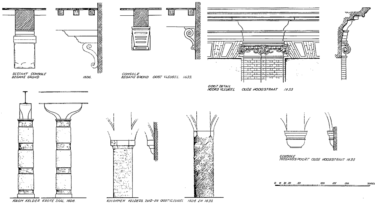
Afb. 5. Amsterdam, het v.m. Oost-Indisch huis, Oude Hoogstraat 24. Opmeting van enige details waaronder het restant van een der grote consoles op de begane grond van de zuidvleugel (tekening J.J. Jehee in 1978).
