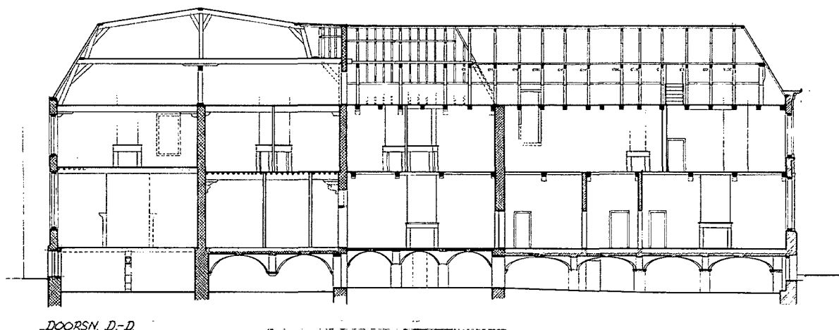
Afb. 8. Amsterdam, het v.m. Oost-Indisch huis, Oude Hoogstraat 24. Dwarsdoorsnede in westelijke richting over de zuidvleugel (links) en de lengte doorsnede over de west vleugel. Proeve van een reconstructie van de bestaande toestand in 1890 naar opmeting van het architectuurbureau Bart van Kasteel en J. Schipper in 1975 en tekeningen van C.H. Peeters in 1890 (tekening J.J. Jehée 1978).
