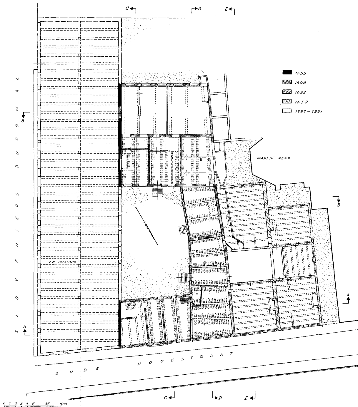
Afb. 3. Amsterdam, het v.m. Oost-Indisch huis, Oude Hoogstraat 24. Plattegrond van de begane grond. Proeve van een reconstructie van de bestaande toestand in 1890 naar opmeting van het architectenbureau Bart van Kasteel en J. Schipper in 1975 en tekeningen van C.H. Peeters in 1890 (tekening J.J. Jehee 1978).
