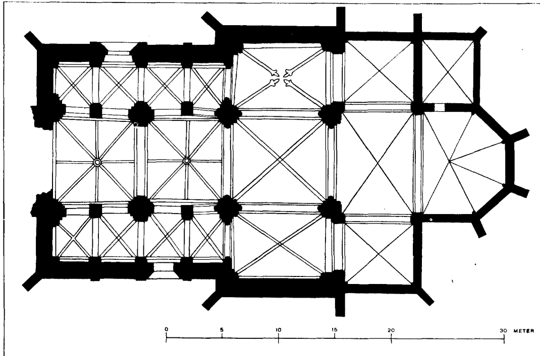
Afb. 5. Plattegrond van de H.H. Simon- en Judas-Kerk te Ootmarsum.
