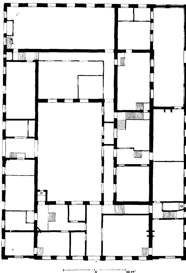
Afb. 62. Plattegrond van het Residentiehuis aan den Haarlemmerdijk (tegenwoordige toestand).
