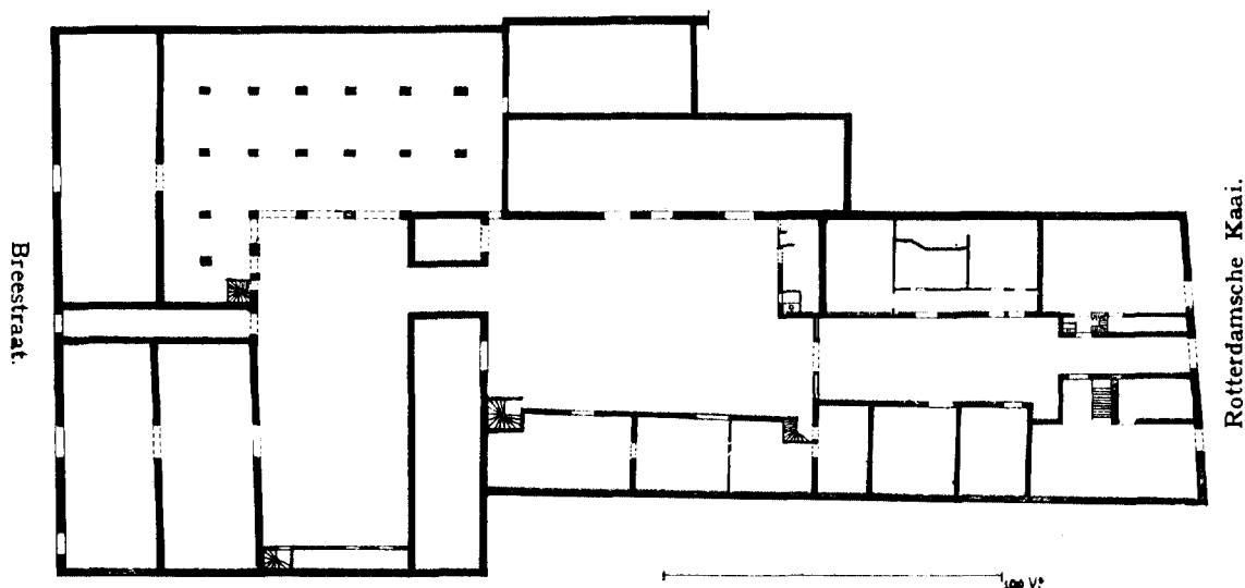
Afb. 22. Plattegrond van het O. I. huis te Middelburg.
