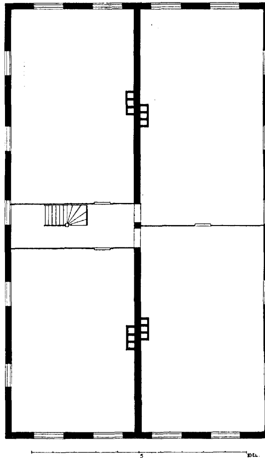
Afb. 50. Plattegrond van de pakhuizen aan de Modderbakken, ingericht tot hospitaal.
