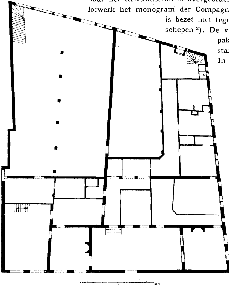
Afb. 74. Plattegrond van het West-Indisch huis aan den IJ-kant.
