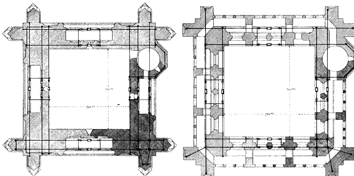
Plattegrond verankering. A.
