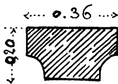
Fig. 4. | Dwarsgordel - en arcadenboog in doorsnede
