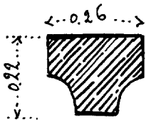
Fig. 3. | Diagonaalrib. (doorsnede)
