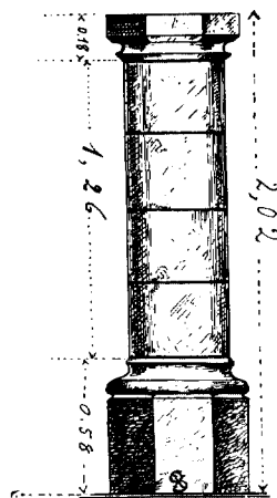
Fig. 6. Kolom. Stadhuis - Hertogmijnch
