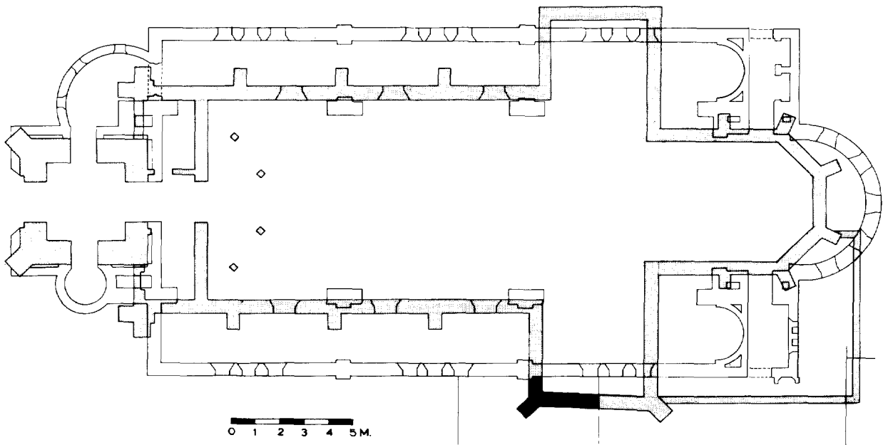
Afb. 4. Berkel-Enschot. Willibrorduskapel. De in 1910 gesloopte kerk (met in zwart aangegeven de onderzochte fundering) ten opzichte van de nieuwbouw van 1910 (tekening F. de Wolf, afd. archeologie Tilburg).
