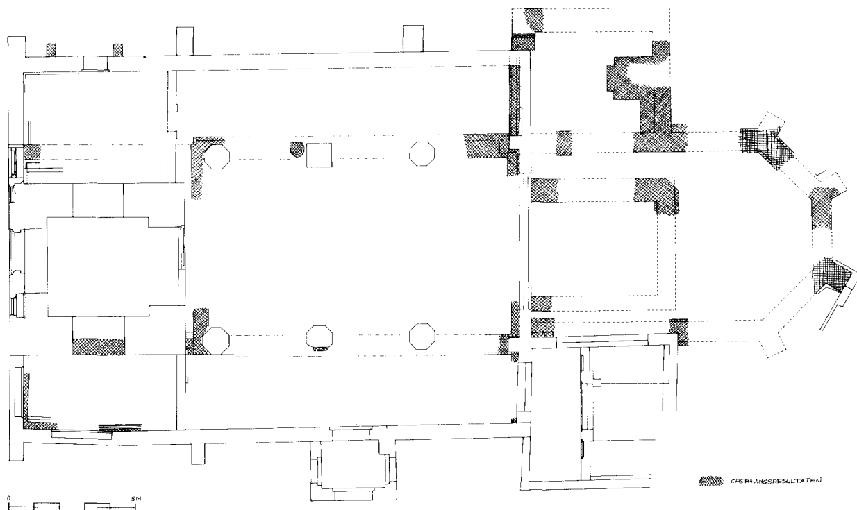
Afb. 3. Plattegrond van NH kerk te Batenburg (G.). Gestippelde lijnen: reconstructie; gearceerde lijnen: opgegraven gedeelten (tekening auteur).
